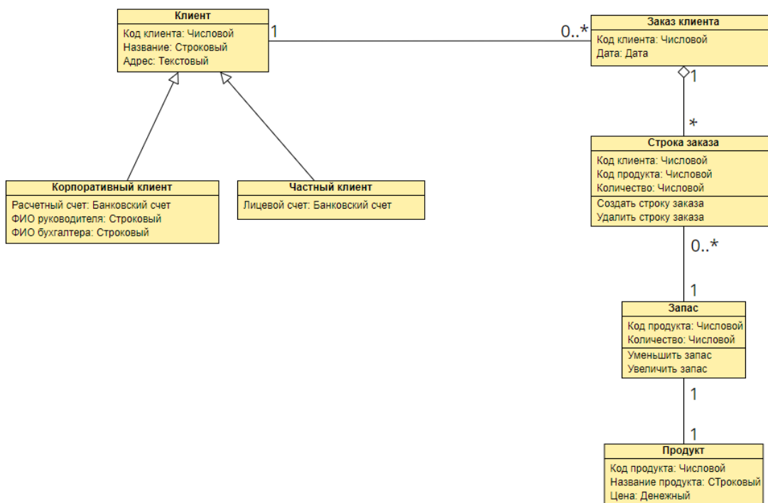
Рис. 1. Диаграмма класса подсистемы учета заказов клиента онлайн-магазина продуктов
